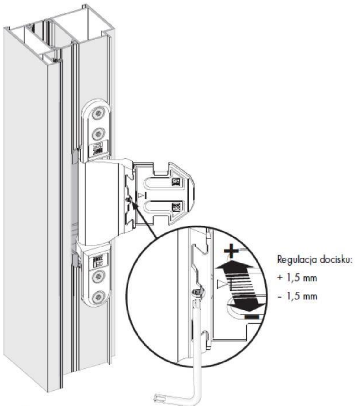
rys. 2: Regulacja zawiasu
