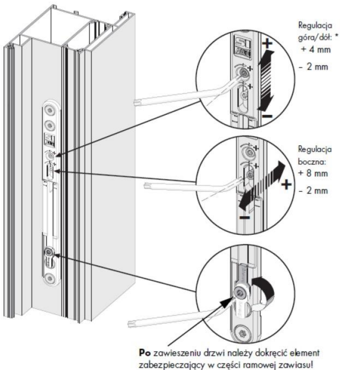
rys. 1: Regulacja zawiasu
