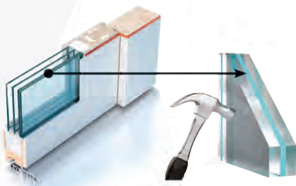
Wkład 3-szybowy z P-2, szkło antywłamaniowe + folie (dwie tafle szkła float + 2 folie) + ciepła ramka przyszybowa
